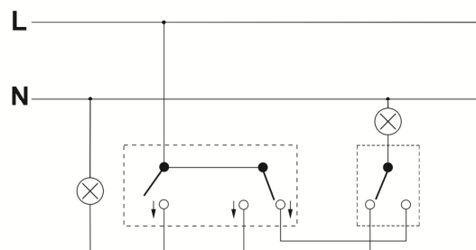
Łącznik jednobiegunowy ze schodowym
