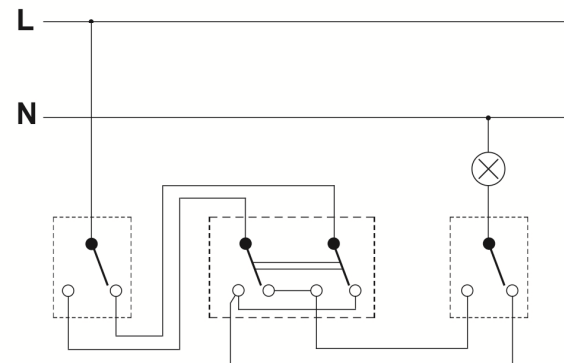
Łącznik krzyżowy ze schodowym
