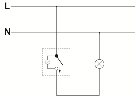
Łącznik jednobiegunowy z podświetleniem
