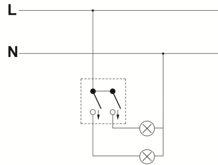
Łącznik świecznikowy
