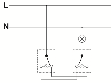
Łącznik schodowy z podświetleniem
