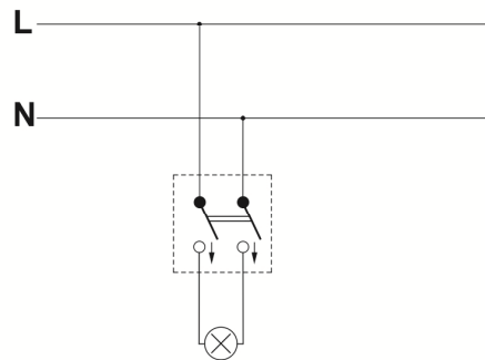
Łącznik dwubiegunowy
