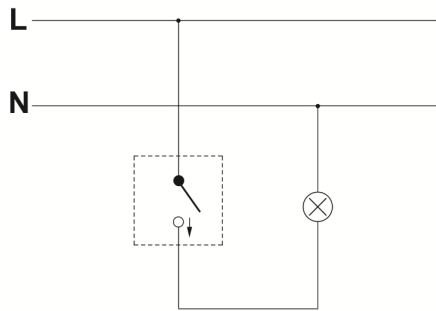
Łącznik jednobiegunowy
