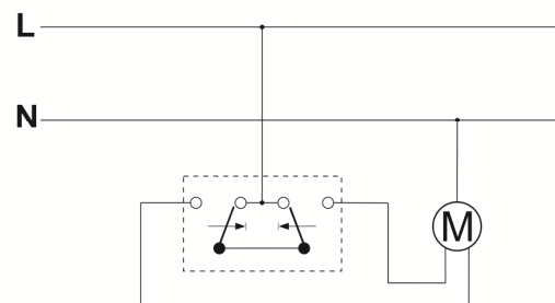
Łącznik żaluzjowy
