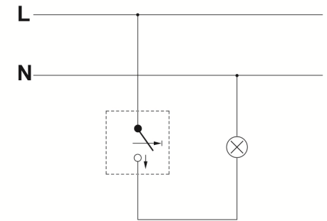
Łącznik zwierny (dzwonek, światło)
