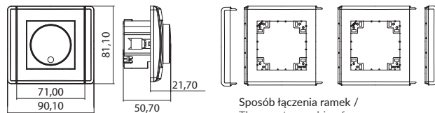
Sposób łączenia ramek / The way to combine frames
