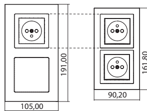
Porównanie ramki DECOvac z ramką uniwersalną podwójną DECO. / Comparison of a DECOvac frame with a double universal frame DECO.
