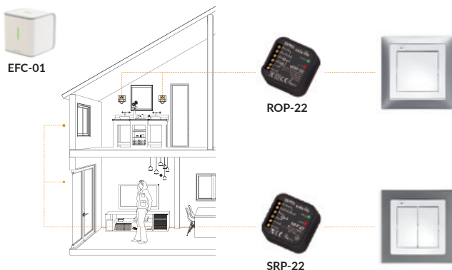
Przykład zastosowania systemu Extra Life. / Extra Life application example.
