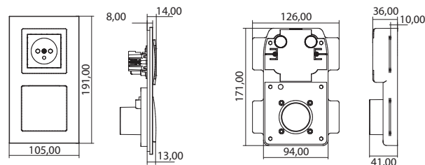
Porównanie ramki DECOvac z ramką uniwersalną podwójną DECO. / Comparison of a DECOvac frame with a double universal frame DECO.
