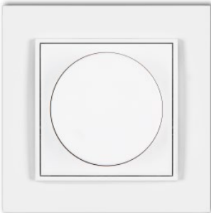
ramka kwadratowa biała / white square frame mechanizm elektronicznego regulatora oświetlenia przyciskowo-obrotowego do współpracy z zasilaczami sterowanymi napięciem 1–10 V biały / white electronic dimmer push-rotary mechanism for use with 1-10V voltage-controlled power supply unit
