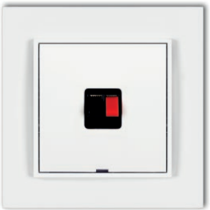
ramka kwadratowa biała / white square frame mechanizm gniazda głośnikowego pojedynczego (2,5 mm 2 ), bez pola opisowego biały / white single loudspeaker socket (2,5 mm 2 ) mechanism, without description field
